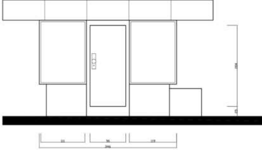
hr.fleischer's Kiosk RÜCKSEITE
