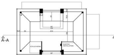
hr.fleischer's Kiosk GRUNDRIß
